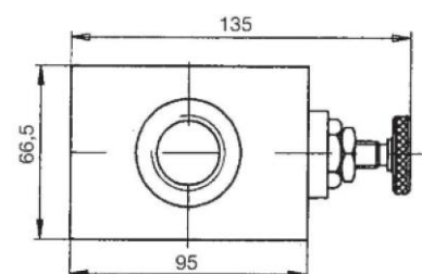
KPP10/...TB(G) Con pilotaje hidráulico
