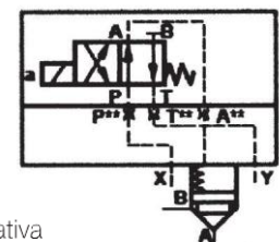
Válvula direccional
