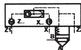
Válvula alternativa
