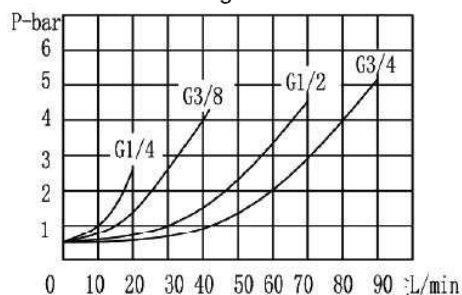
Pérdida de carga
