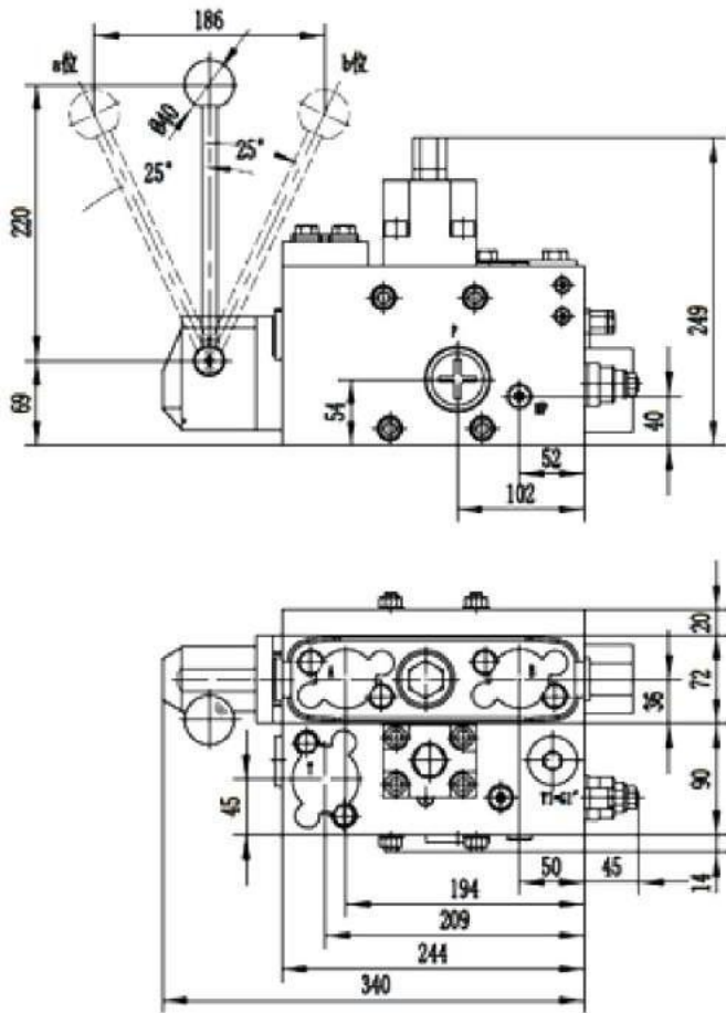
Estructura General
