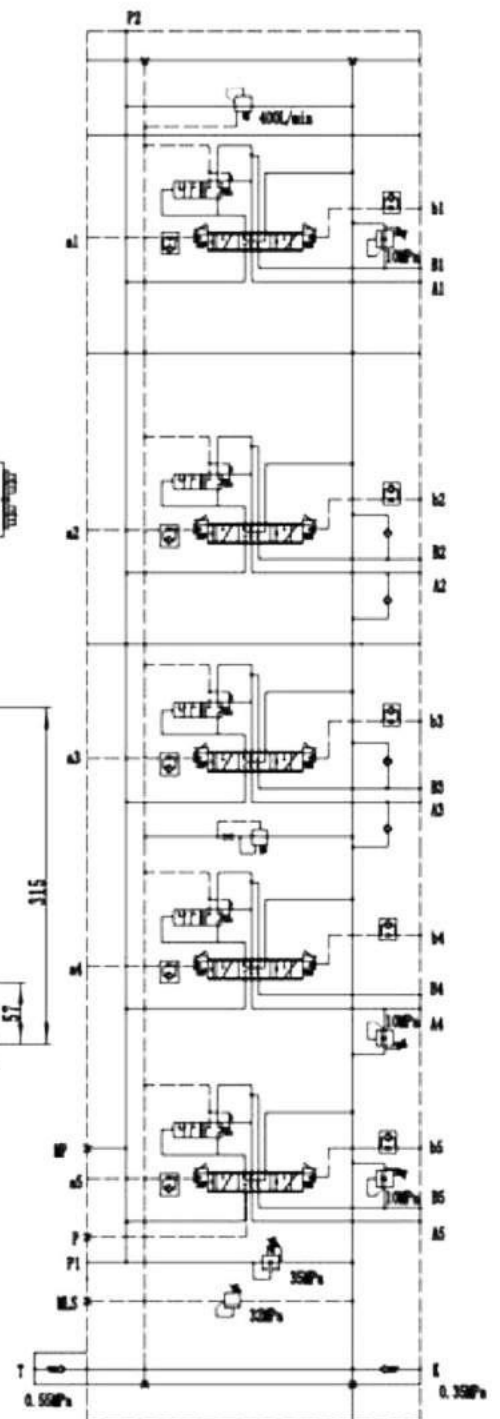
Esquema Hidráulico
