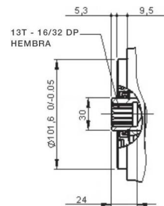
Brida de fijación para bomba TANDEM
