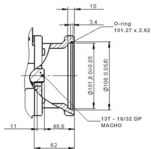
Brida de fijación SAE B
