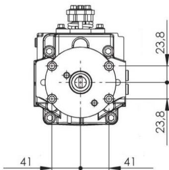
Brida trasera Bosch GR 1
