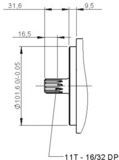
Eje estriado Z11 16/32 DP
