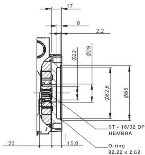
Brida de fijación SAE A
