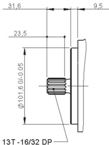
Eje estriado Z13 16/32 DP
