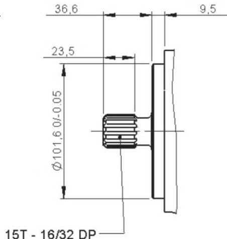
Eje estriado Z15 16/32 DP
