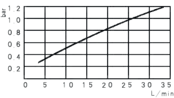
Caída de presión
