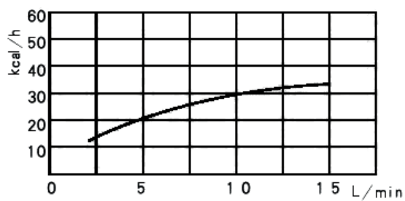
Potencia de enfriamiento
