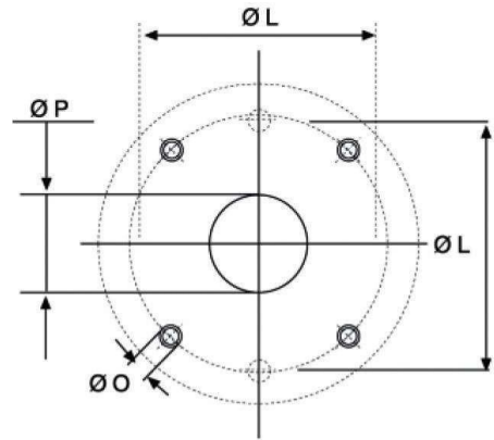
Montaje 2 agujeros
