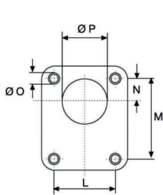
Montaje rectangular 4 agujeros
